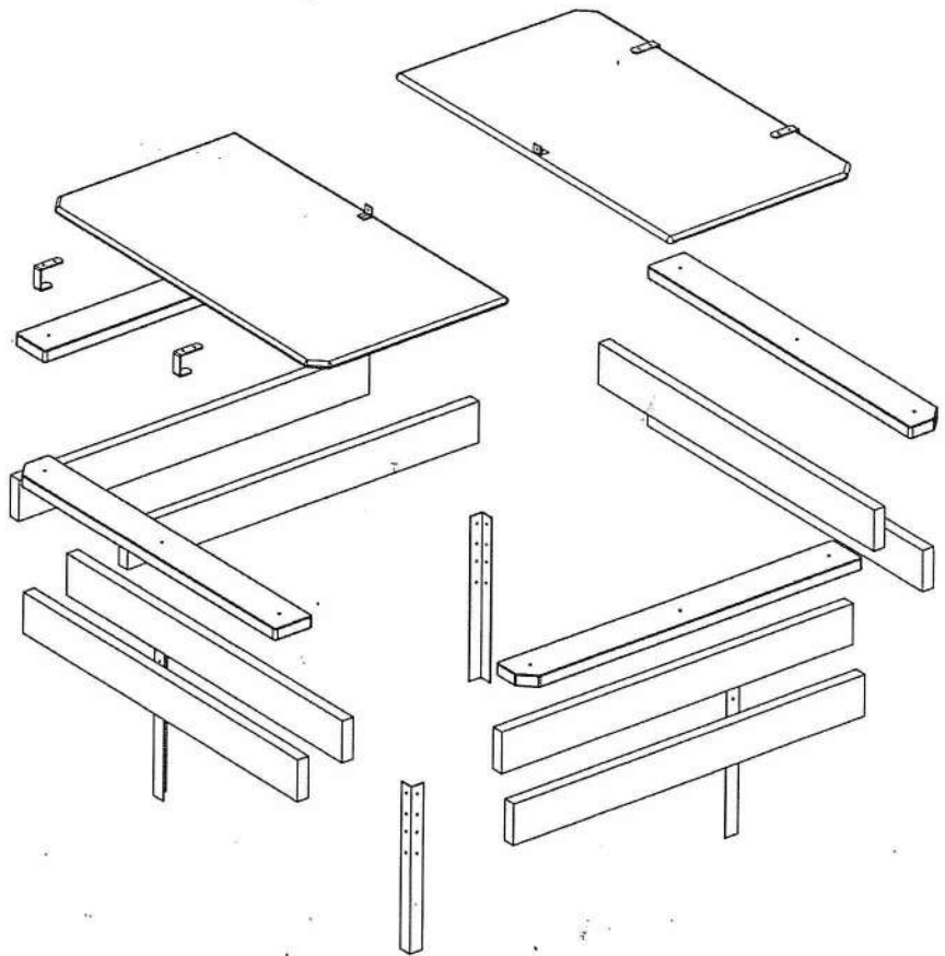
Slide assembling sandbox (Схема сборки песочницы)
